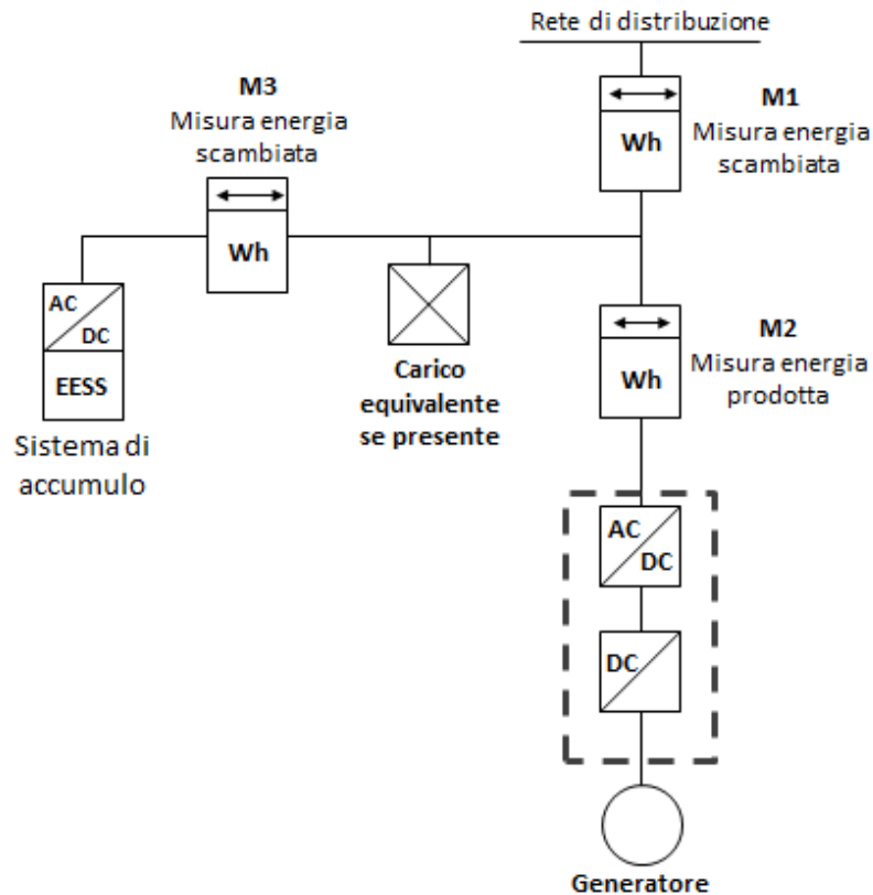
Figura 43 – Misura dei flussi di energia con accumulo posizionato nella parte d’impianto in corrente alternata a monte del contatore dell’energia generata
