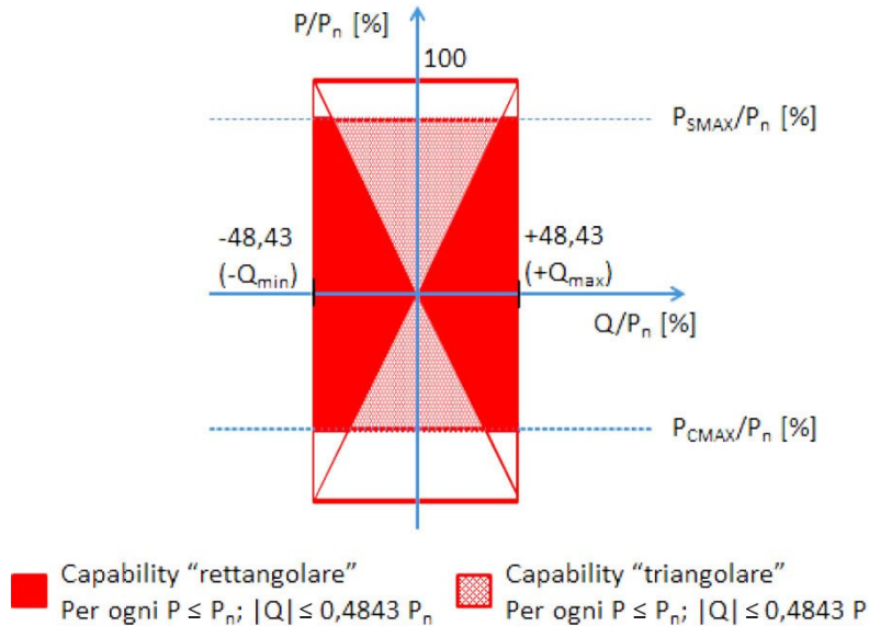
Figura 62 – Capability per un sistema di accumulo con inverter bidirezionale
