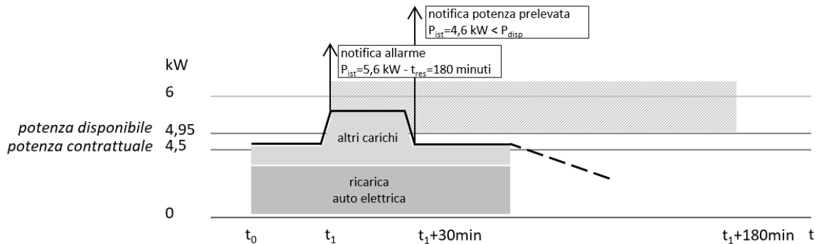
Figura 98 Figura X3 – Esempificazione dell’invio di segnali provenienti dal misuratore intelligente 2G M1 sul canale Chain 2 durante l’evento di superamento della potenza disponibile
