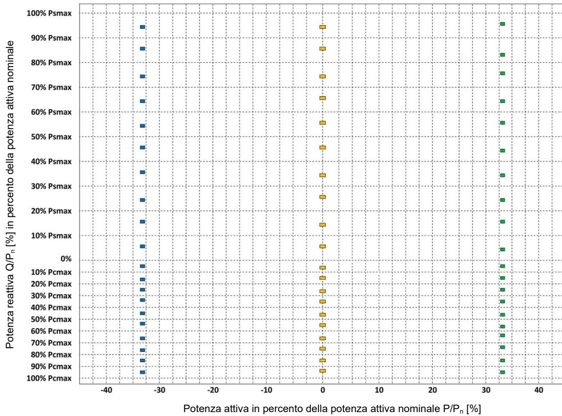
Figura 63 – Esempio di Grafico P(Q). Massima potenza reattiva induttiva e capacitativa erogata in funzione della potenza attiva (qui è rappresentato il caso di un sistema di accumulo di potenza fino a 11,08 kW, che deve poter erogare con un \cos\phi = 0,95 , ovvero Q_{min}/P_n = 0,3286 )
