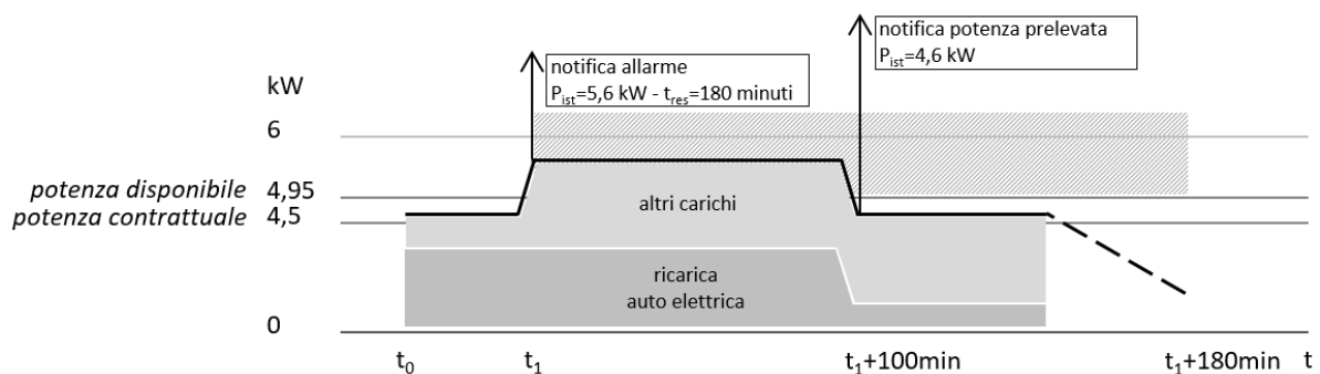
Figura 99 Figura X4 – Esempificazione dell’invio di segnali provenienti dal misuratore intelligente 2G M1 sul canale Chain 2 durante l’evento di superamento della potenza disponibile e successivo intervento della funzione di power management presente nel CIR
