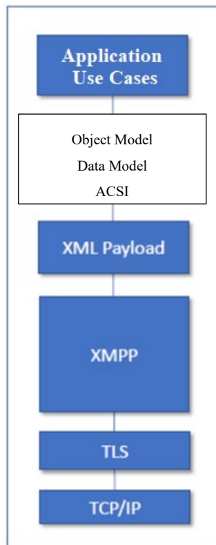
Figura 100 Figura X5– Pila protocollare per il protocollo di comunicazione CIR-RO.
