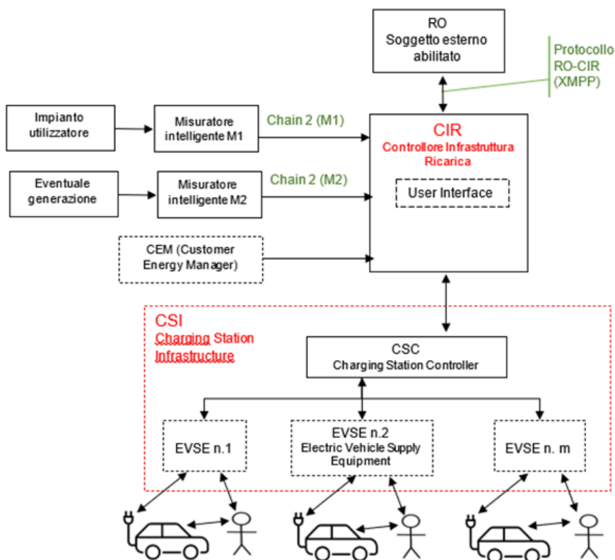
Figura 96 Figura X1– Architettura di riferimento per le interfacce di comunicazione del CIR
