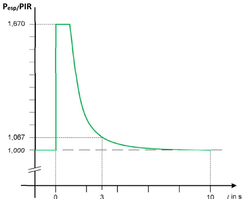
Figura 4- Curva limite di immissione
