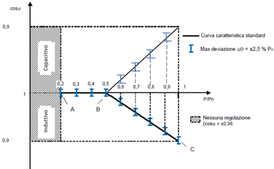
Figura 50 – Curva caratteristica standard \cos\phi = f(P)
