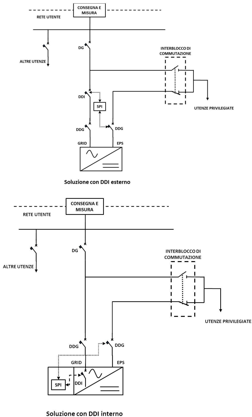
Figura 19 – Esempio di sistema di produzione di energia con funzionamento in isola attraverso porta dedicata (DDI esterno e DDI interno)
