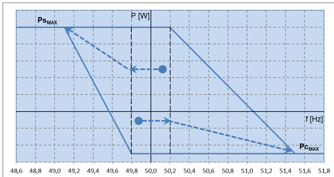
Figura 31 – Regolazione della potenza attiva in condizioni di sovra e sottofrequenza
